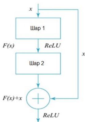
Рис. 1. Залишковий блок архітектури ResNet
