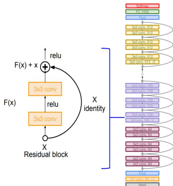
Рис. 2. Залишковий блок архітектури ResNet
